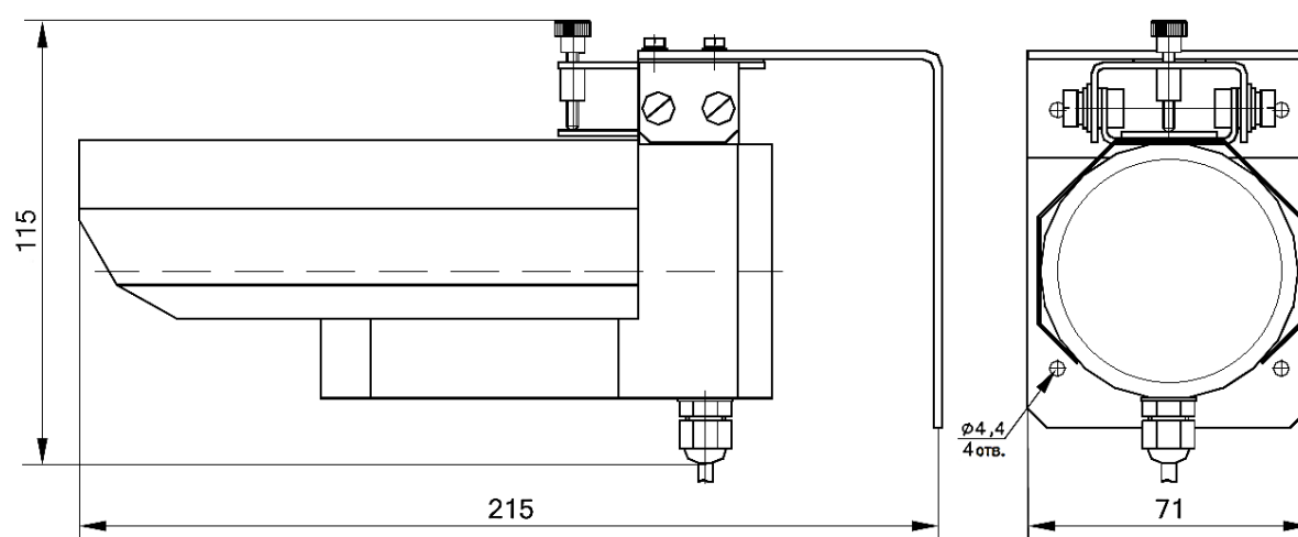
Рисунок 1.2 - Габаритный чертеж
